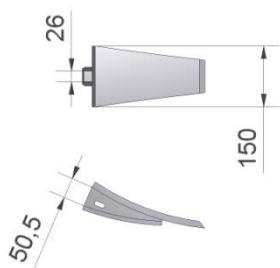
Figuur 18.1.5-Art.nr. 509055 Figuur 18.1.5-Art.nr. 509055A (Mangaan)
