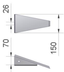
Figuur 6.3.14-Art.nr. 509056 Figuur 6.3.14-Art.nr. 509056A (Mangaan)
