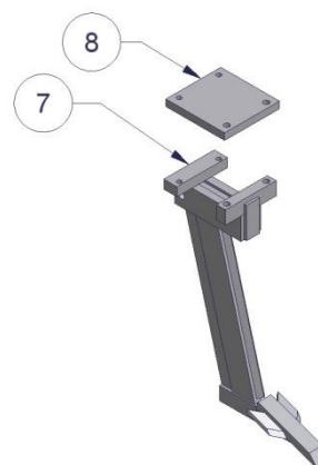
Figuur 18.1.1.4-Flevo tand
