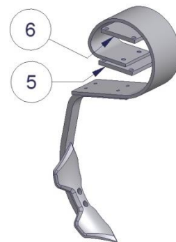
Figuur 6.3.1.5-Tand TBV
