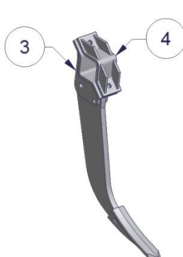
Figuur 18.1.1.2-Tand TSB-R-25
