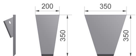
Figuur 18.1.18-Art.nr. 529027 (200mm) Art.nr. 529027A (200mm)(Mangaan) Art.nr. 529028 (350mm) Art.nr. 529028A (350mm)(Mangaan)
