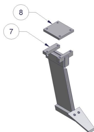
Figuur 18.1.1.4-Rechte tand
