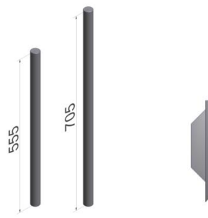
Figuur 18.1.13-Art.nr. 529044 (555mm) Art.nr. 5290442 (705mm)
