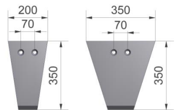
Figuur 18.1.14-Art.nr. 529032 (200mm) Art.nr. 529034 (350mm)
