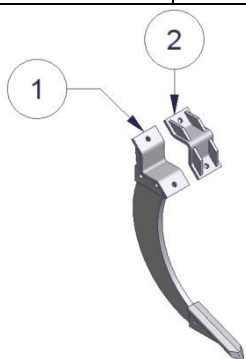
Figuur 18.1.1.1-Tand TSB-20
