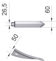
Figuur 6.3.11-Art.nr. 509053 Figuur 6.3.11-Art.nr. 509053A (Mangaan)
