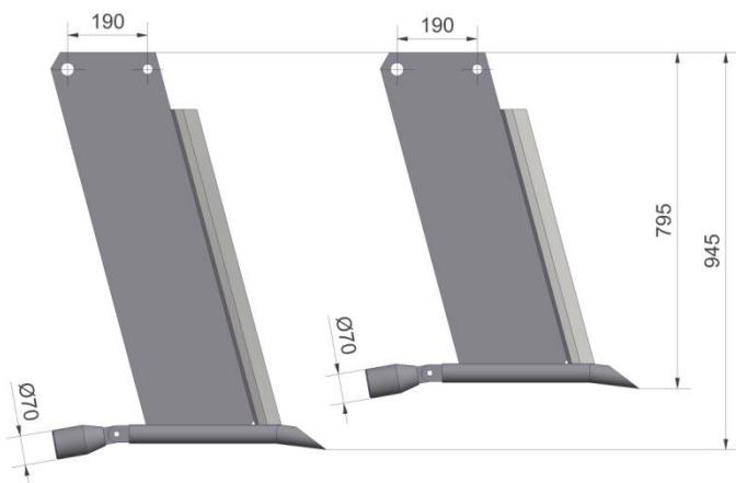
Figuur 18.1.26-Art.nr. 529007 (moltand 795mm) Art.nr. 529008 (moltand 945mm)
