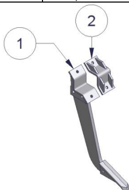
Figuur 18.1.1.1-Tand TSB-R-20
