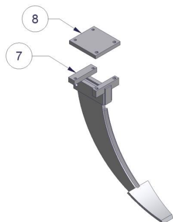
Figuur 18.1.1.4-Gebogen tand
